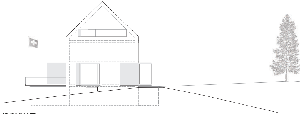
ANSICHT OST 1:200
