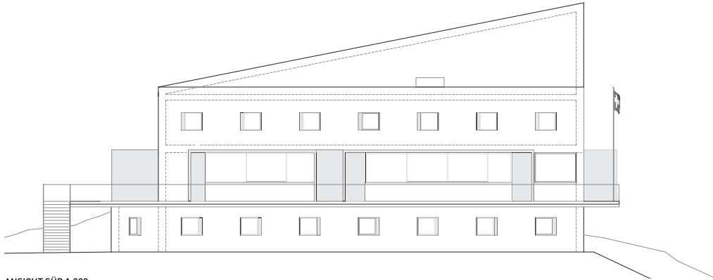
ANSICHT SÜD 1:200
