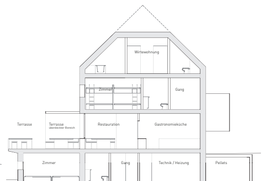
QUERSCHNITT 1:200
