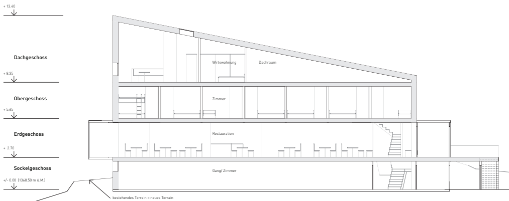
LÄNGSSCHNITT 1:200
