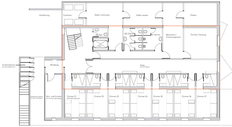
GRUNDRISS SOCKELGESCHOSS 1:200
